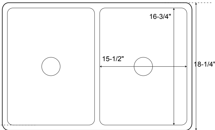
Top
